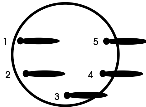
5 Pin Male DIN Plug
